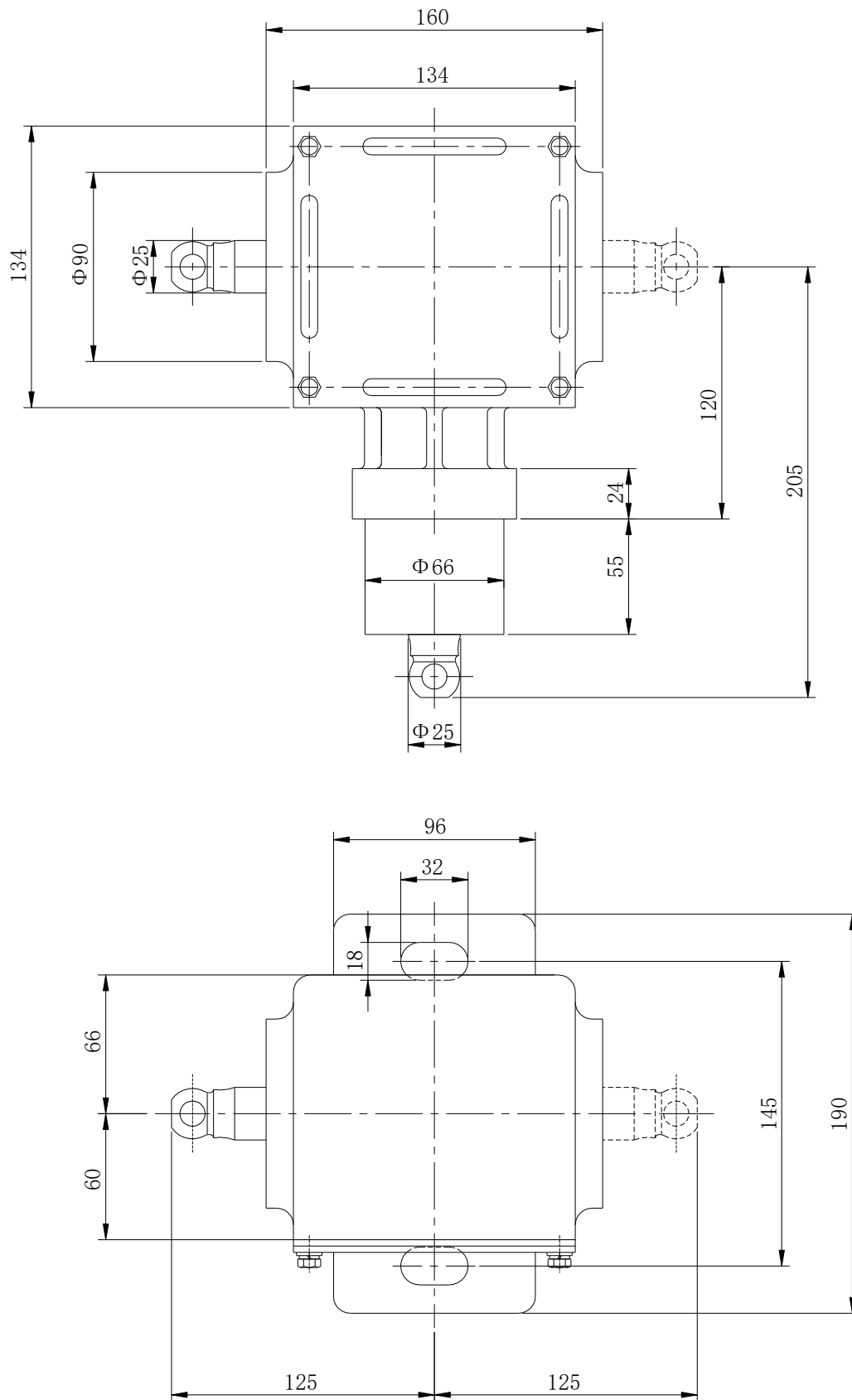
附图 4 换向齿轮盒尺寸图
