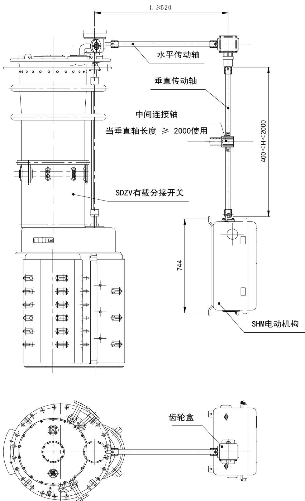
附图 5 SDZV 分接开关与 SHM 电动机构连接布置图
