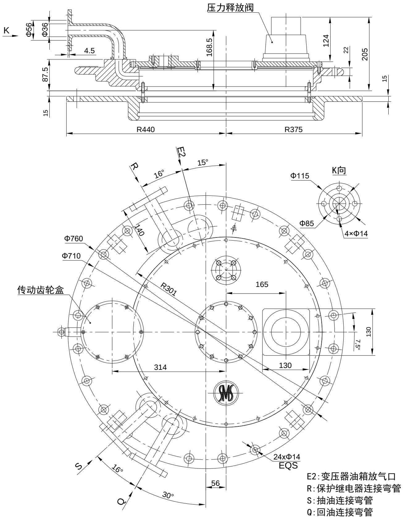
附图 2 SDZV 有载分接开关变压器安装法兰配压力释放尺寸
