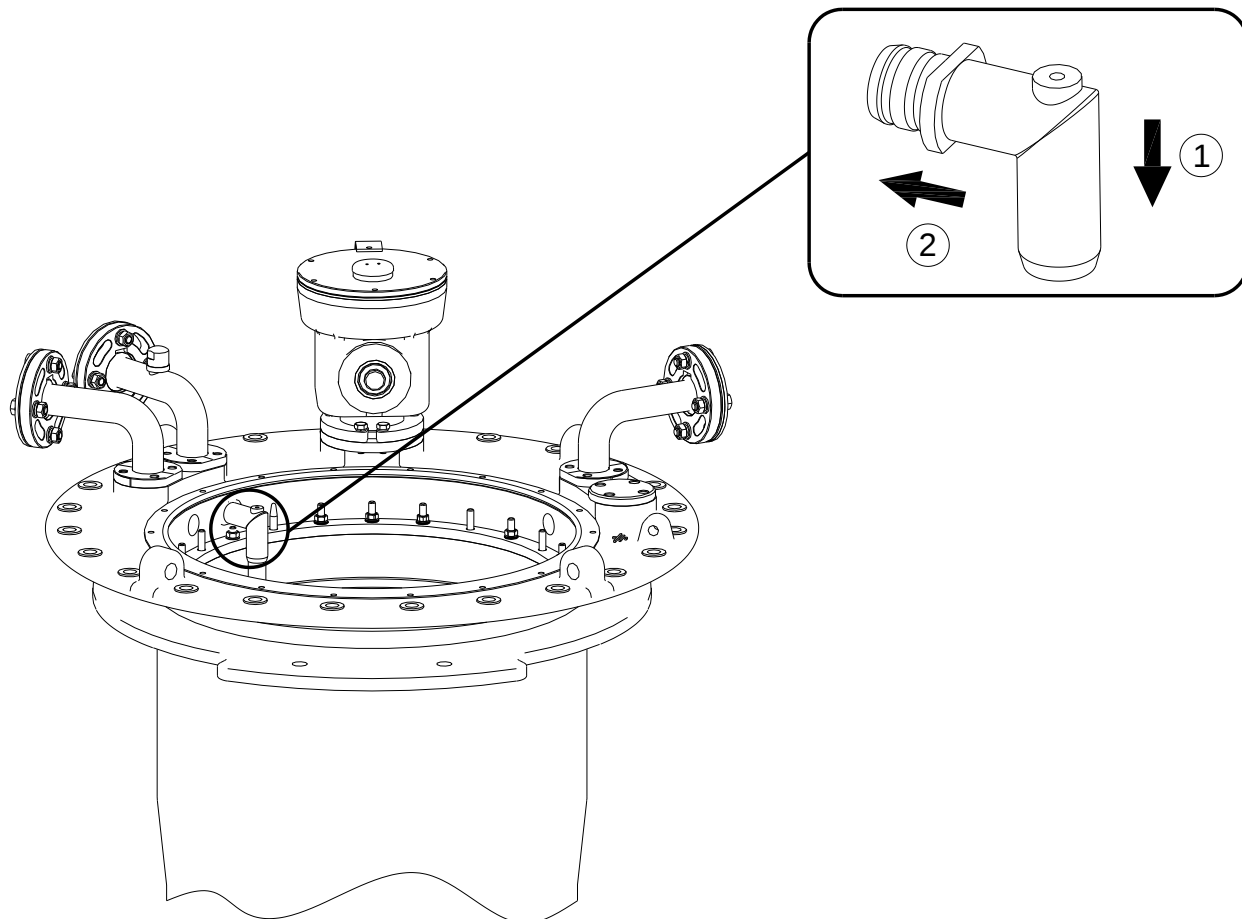
图 5-15 安装抽油管示意图
