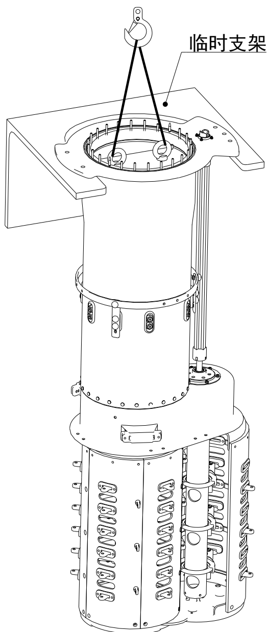
图 5-11 有载分接开关在临时支架上的位置
