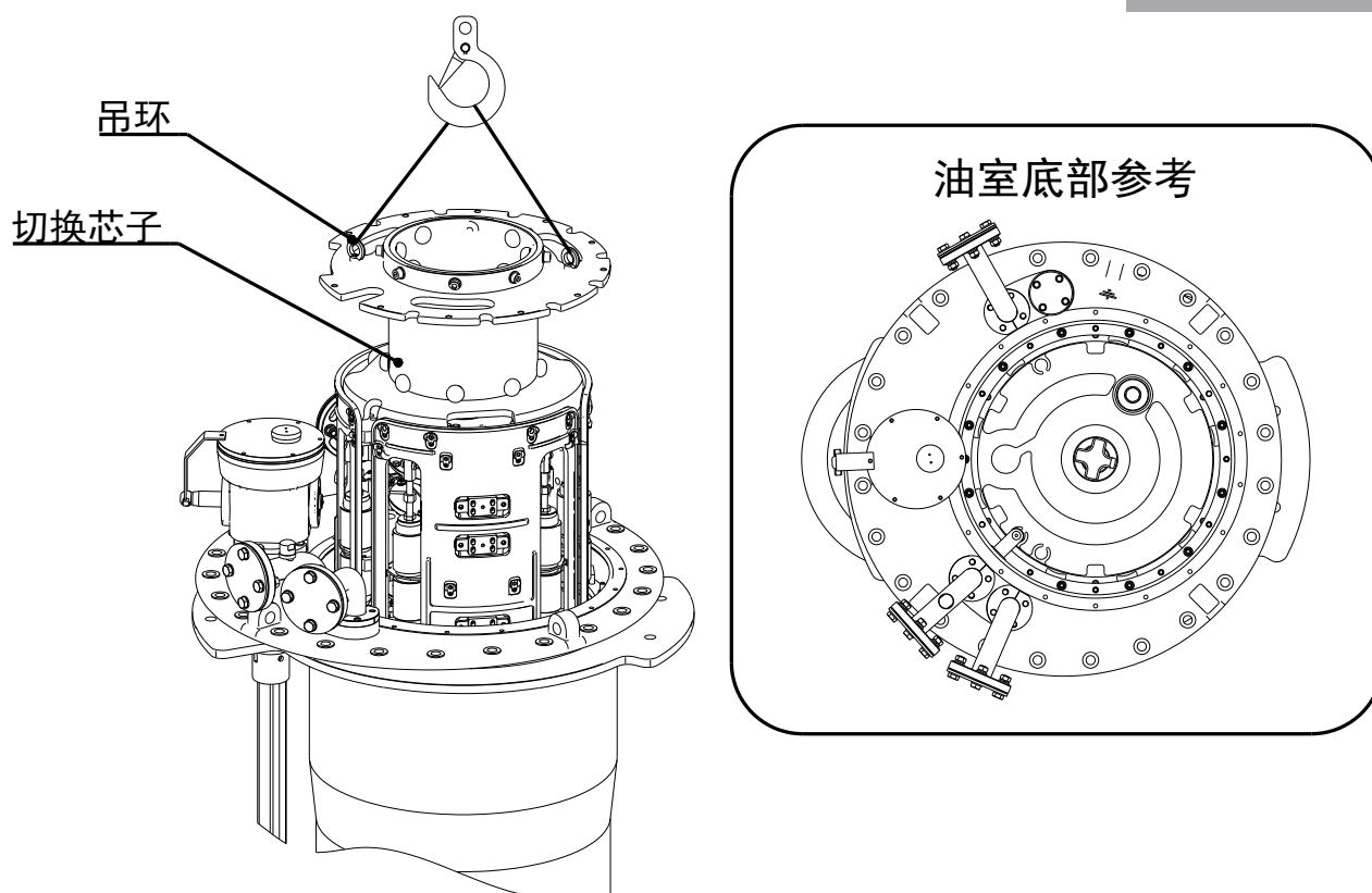
图 5-5 垂直起吊切换开关
