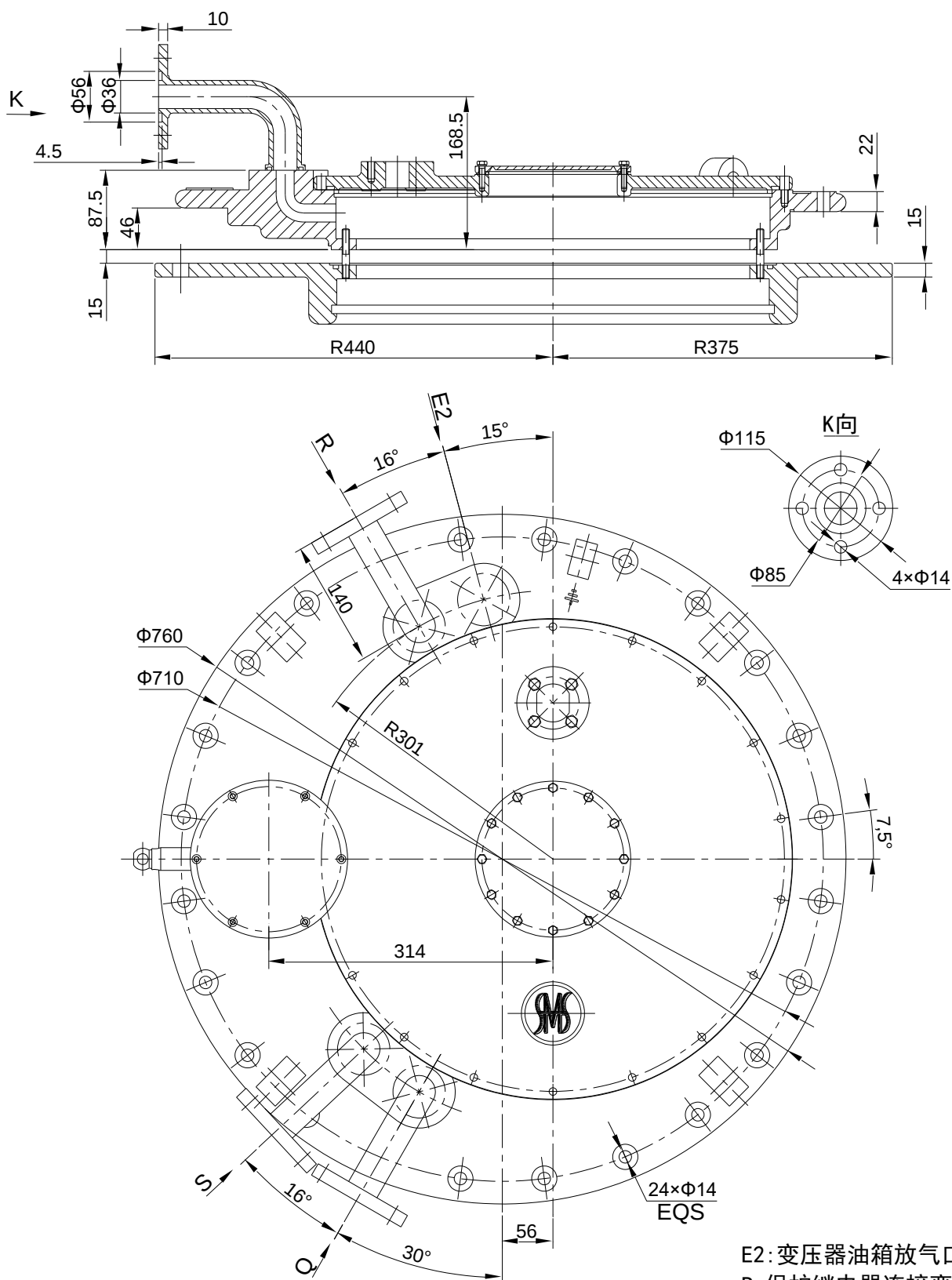
附图 1 SDZV 有载分接开关变压器安装法兰尺寸
