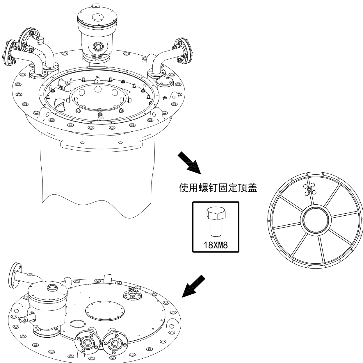
图 5-17 顶盖安装步骤
