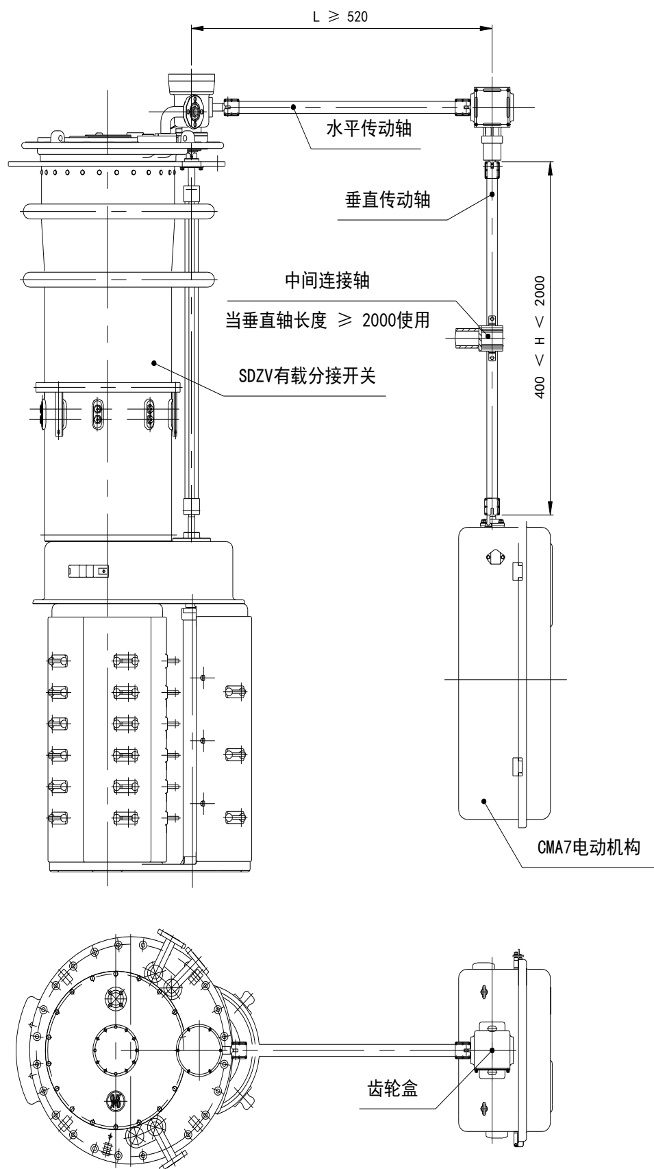
附图 6 SDZV 分接开关与 CMA7 电动机构连接布置图
