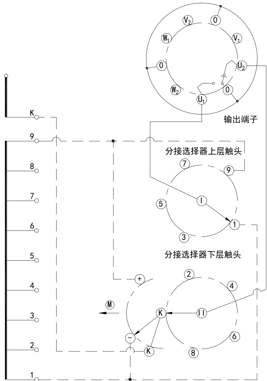
附图 10 SDZV 有载分接开关 10193W 工作位置表和接线原理图
