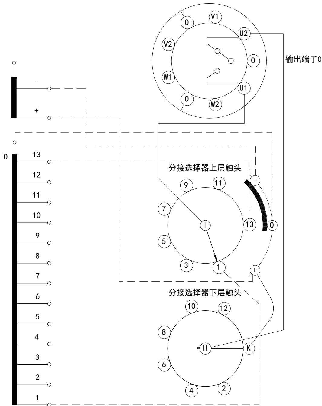
附图 51 VCM 型分接开关工作位置表和接线图 (14271G)
