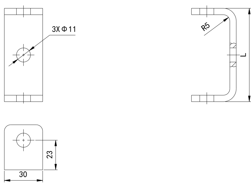
VCM型 I 800触头端子联接图
