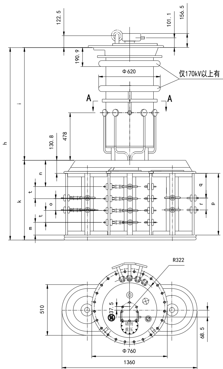
附图 33 VCM I 800 多级分接开关外形尺寸图
