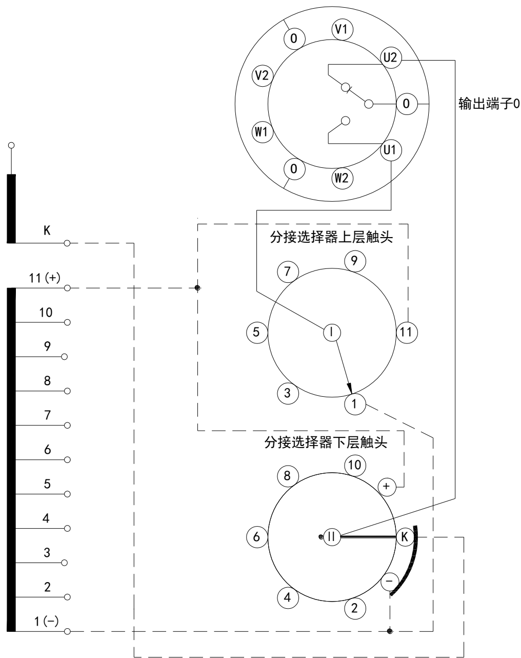
附图 48 VCM 型分接开关工作位置表和接线图 (12233W)
