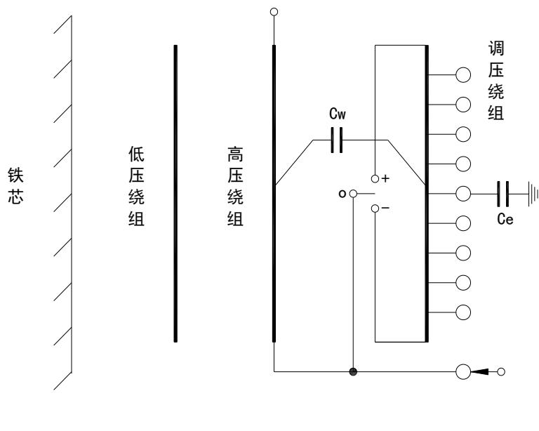
图 5-2 双绕组变压器正反调绕组布置
