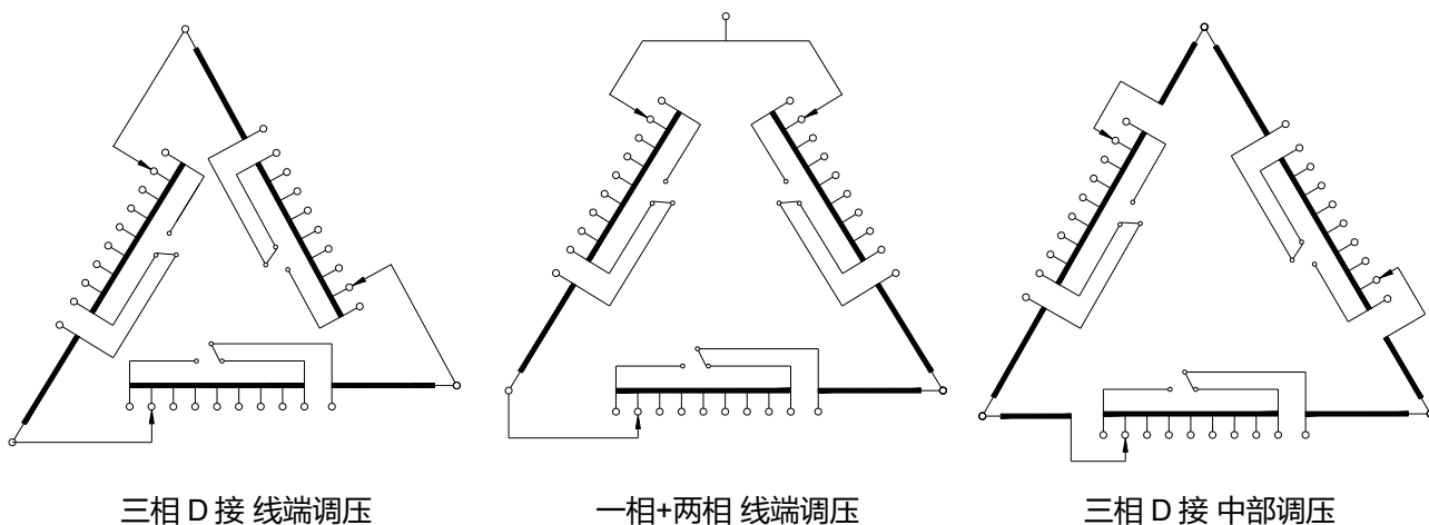
图 5-3 用于 D 接变压器绕组的基本接法
