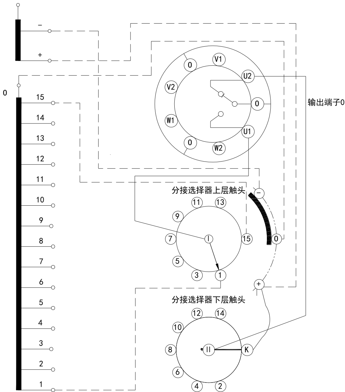
附图 57 VCM 型分接开关工作位置表和接线图 (16311G)
