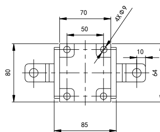
中间支撑盒外型尺寸图
