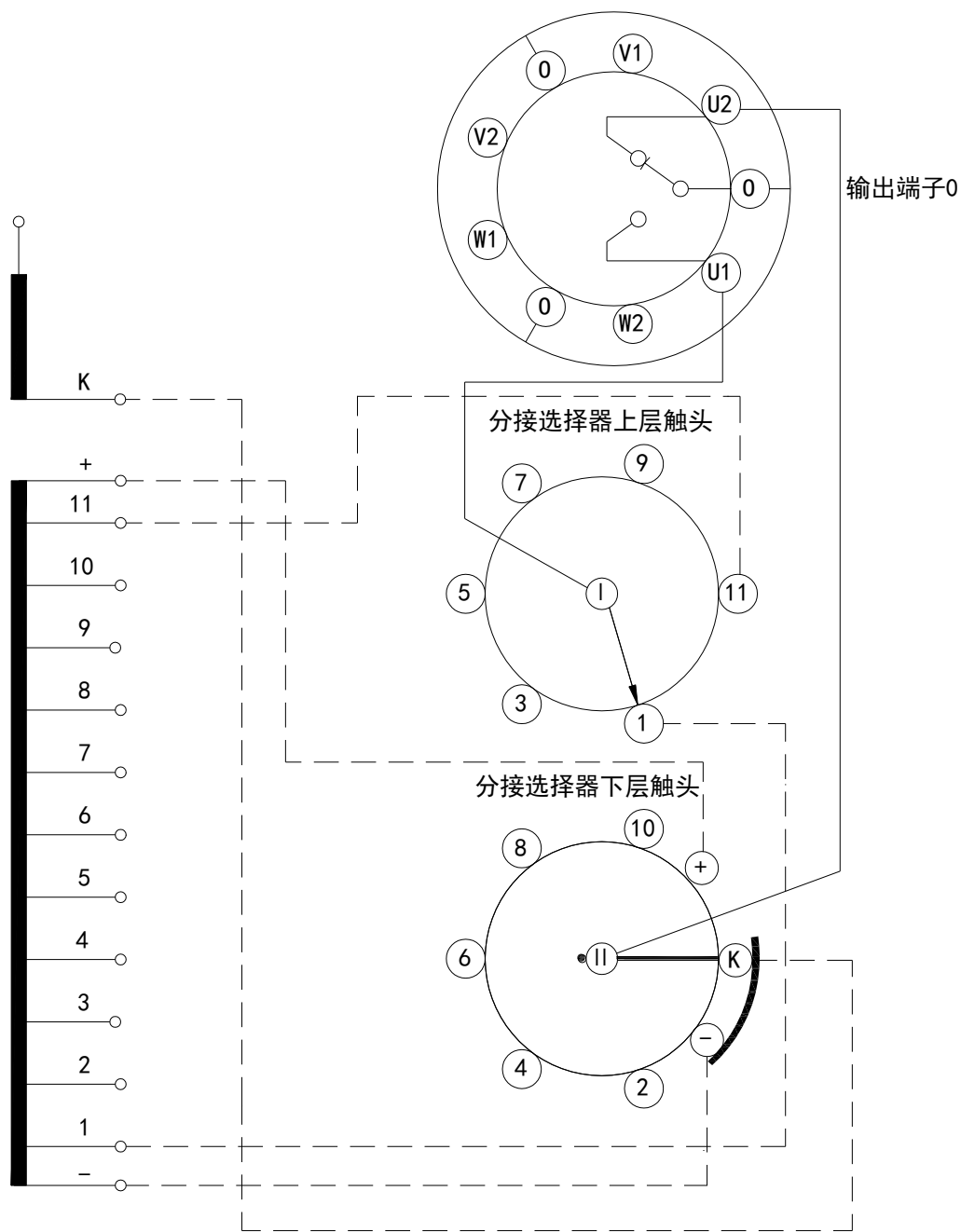
附图 46 VCM 型分接开关工作位置表和接线图 (12231W)
