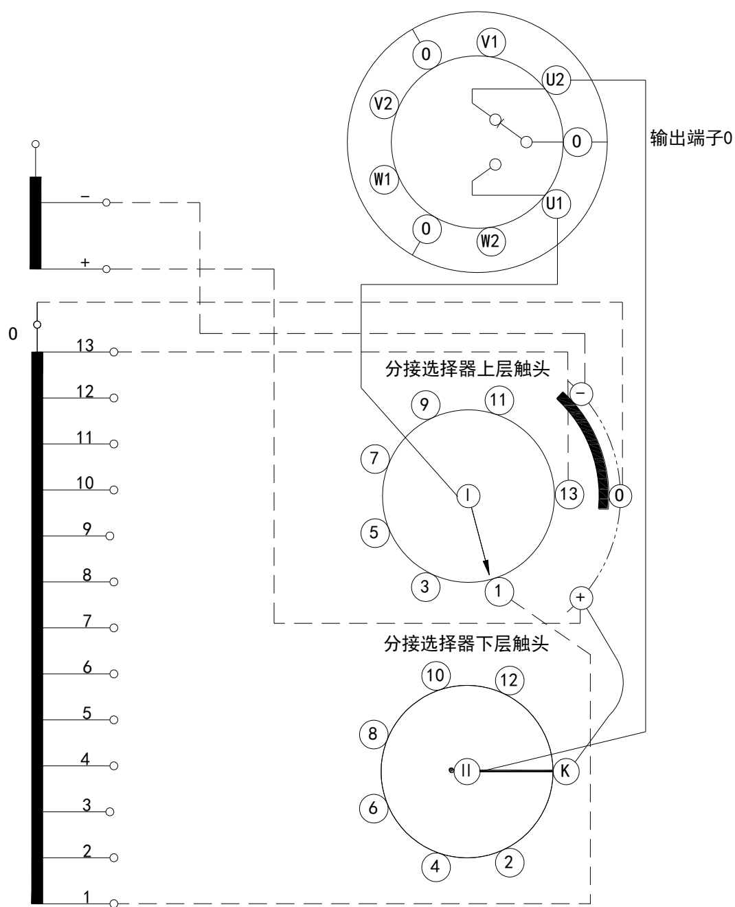
附图 53 VCM 型分接开关工作位置表和接线图 (14273G)
