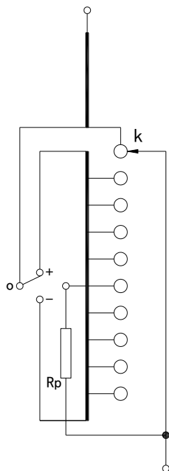
图 5-1 电位电阻恒定连接方式
