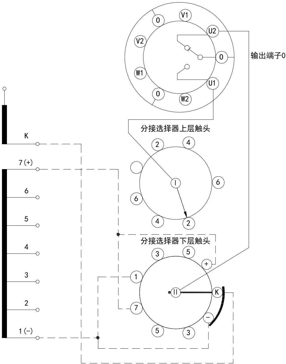
附图 50 VCM 型分接开关工作位置表和接线图 (14131W)
