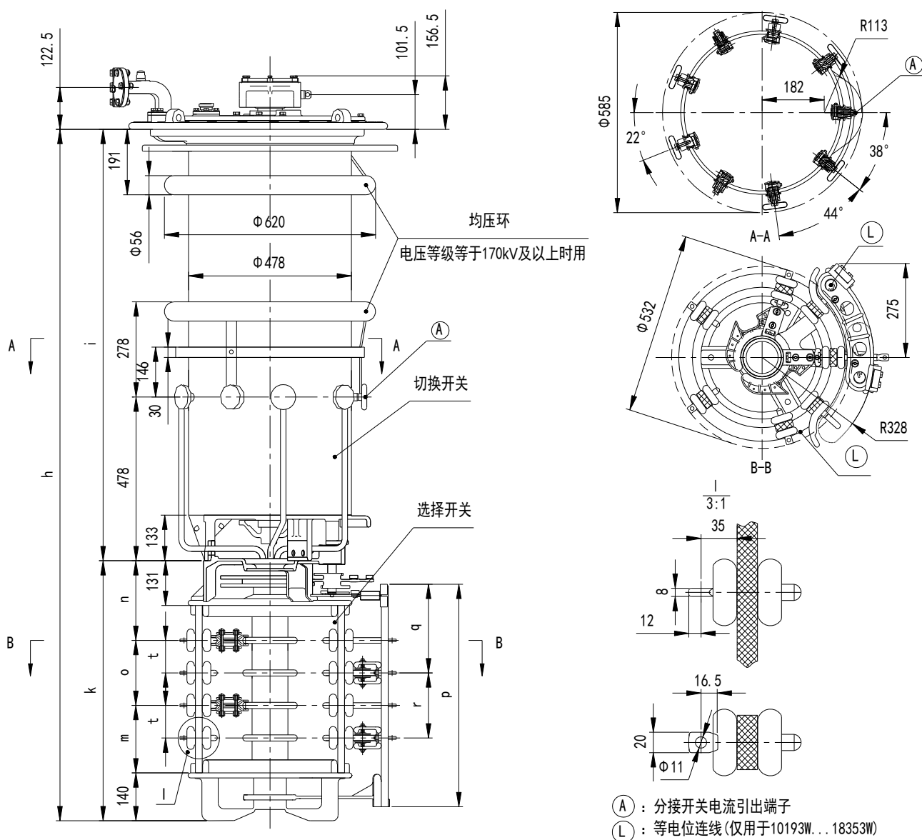
附图 5 VCM 型分接开关 II 500/600 带极性选择器
