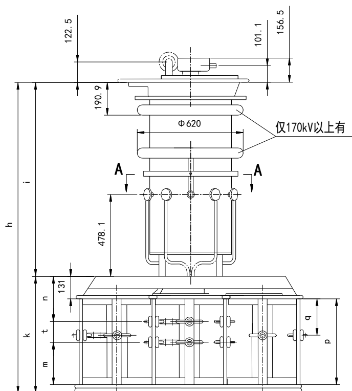
附图 32 VCM I 500/600 多级分接开关外形尺寸图
