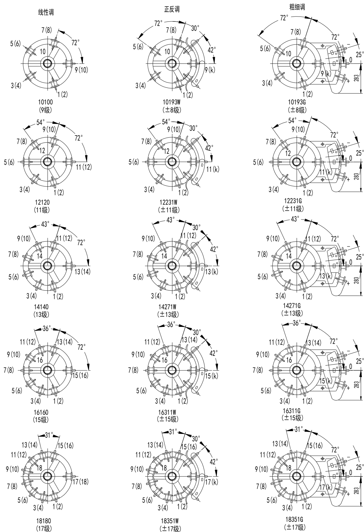
附图 18 VCM 型分接开关触头排列布置示意图
