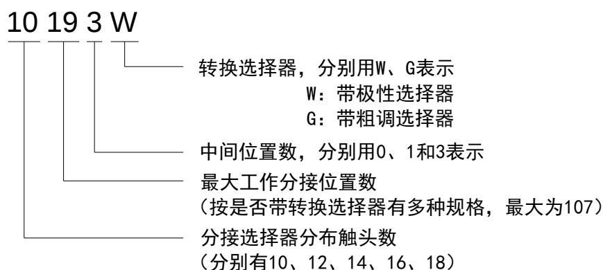
图 3-2 分接选择器基本连接方式说明
