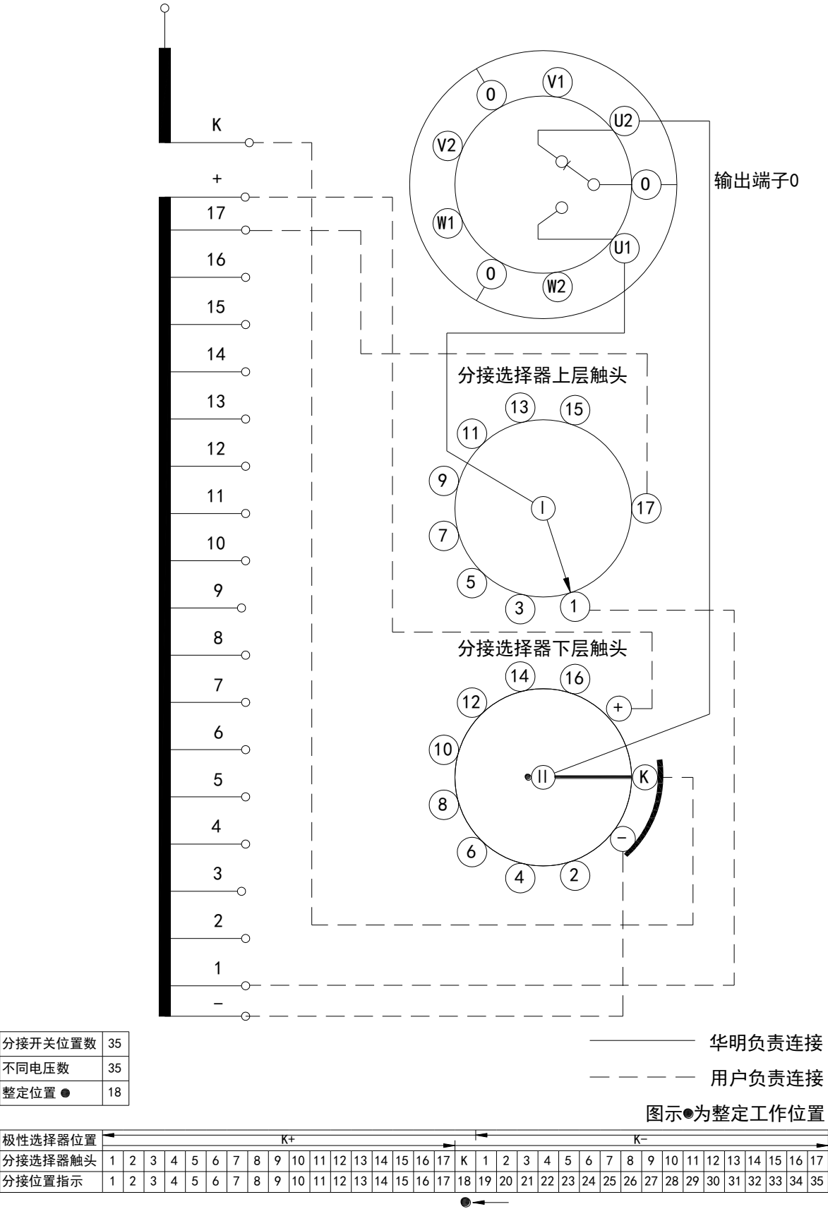
附图 64 VCM 型分接开关工作位置表和接线图 (18351W)
