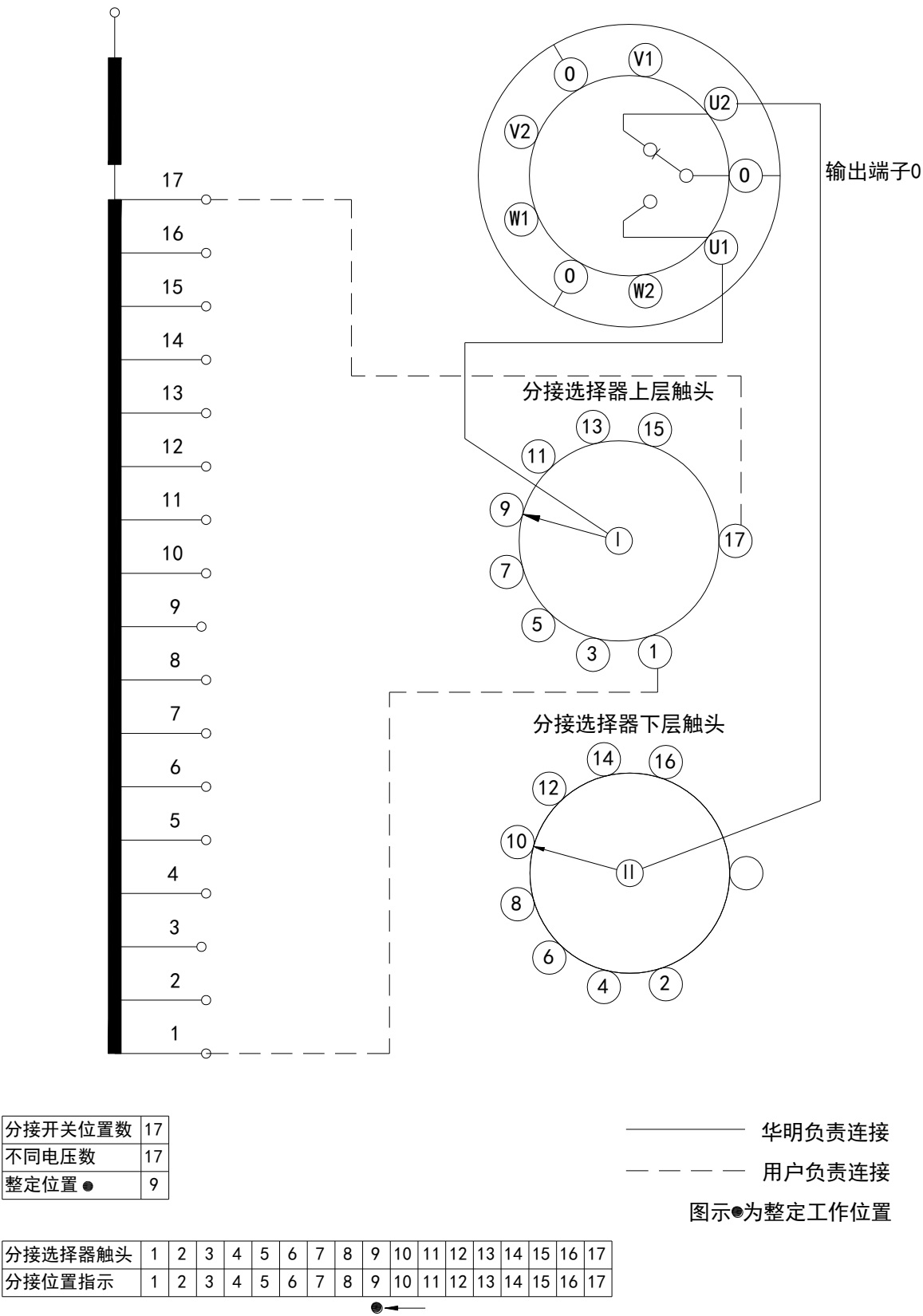
附图 61 VCM 型分接开关工作位置表和接线图 (18170)
