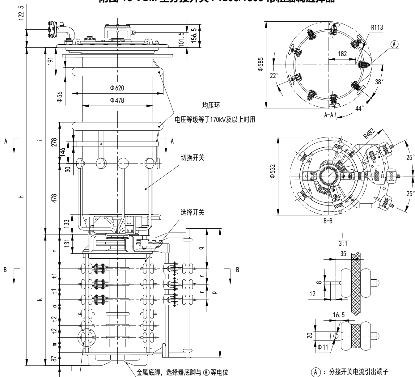
附图 15 VCM 型分接开关 I 1200/1500 带粗细调选择器
