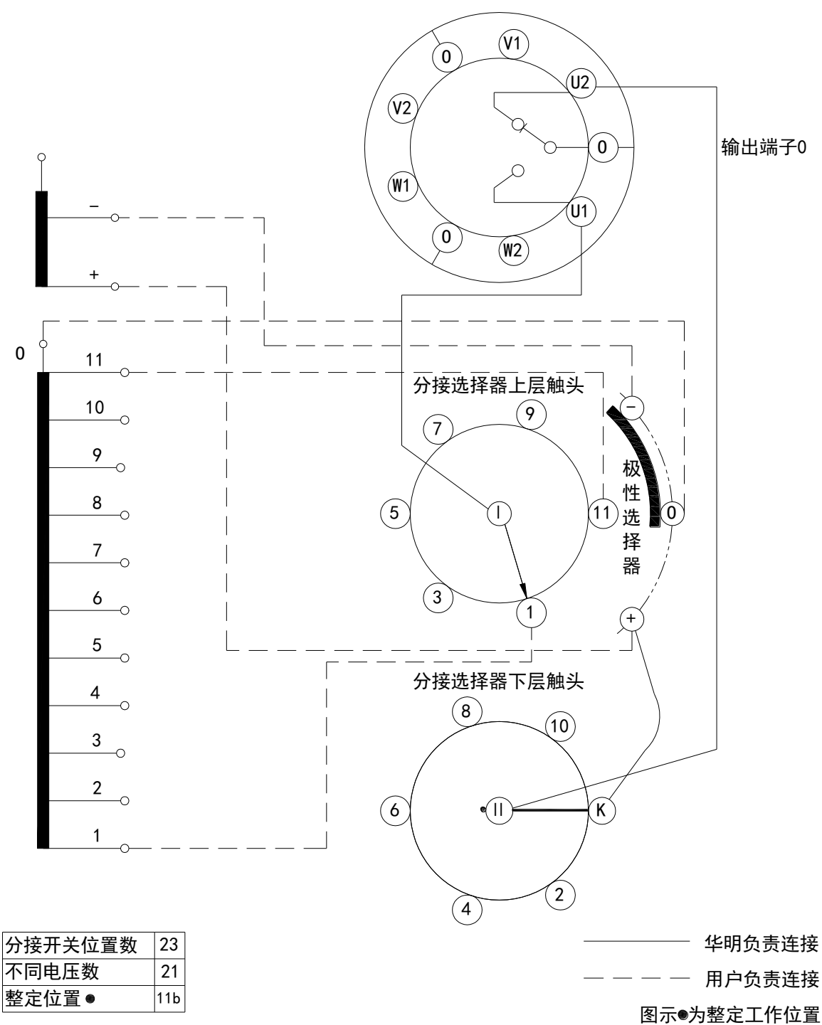
附图 47 VCM 型分接开关工作位置表和接线图 (12233G)
