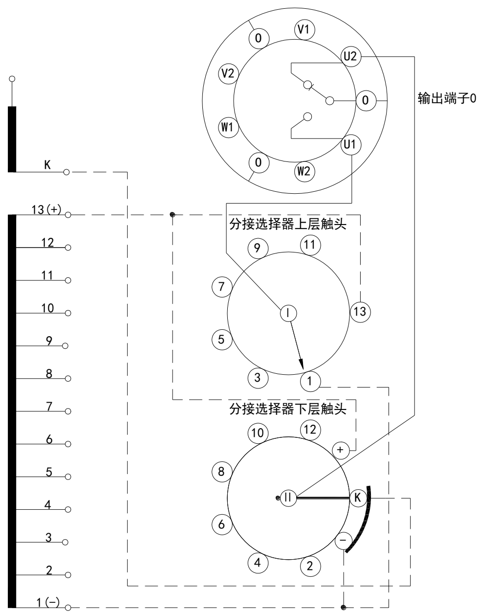
附图 54 VCM 型分接开关工作位置表和接线图 (14273W)
