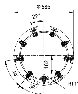
A-A剖视
