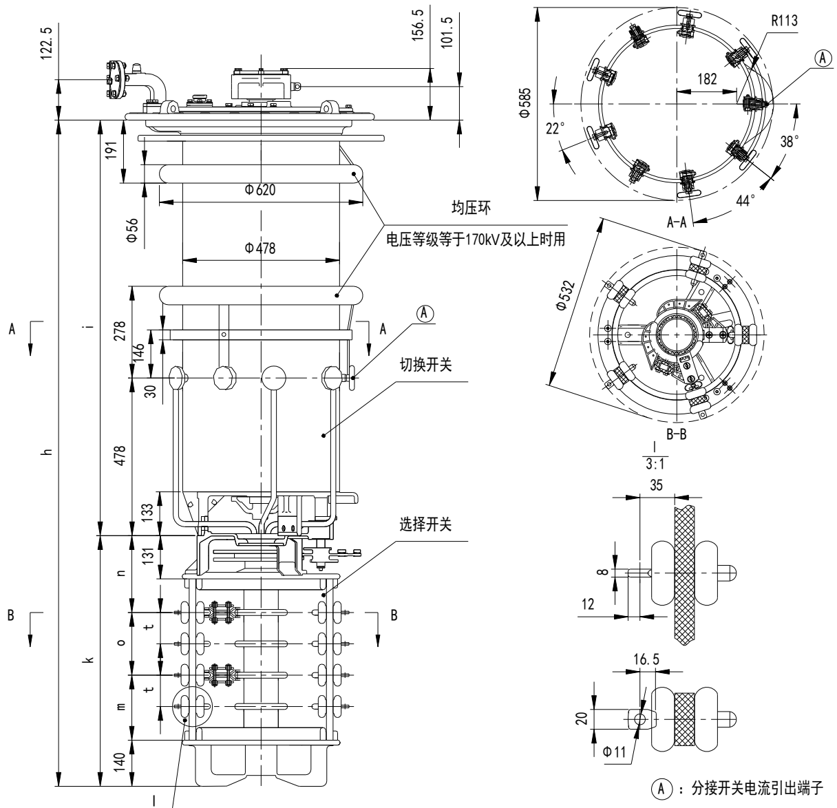
附图 4 VCM 型分接开关 II 500/600 不带极性选择器
