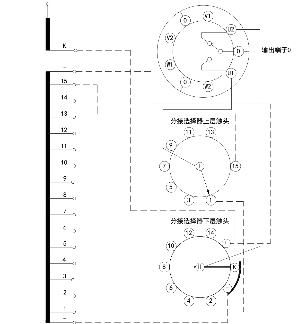
附图 58 VCM 型分接开关工作位置表和接线图 (16311W)
