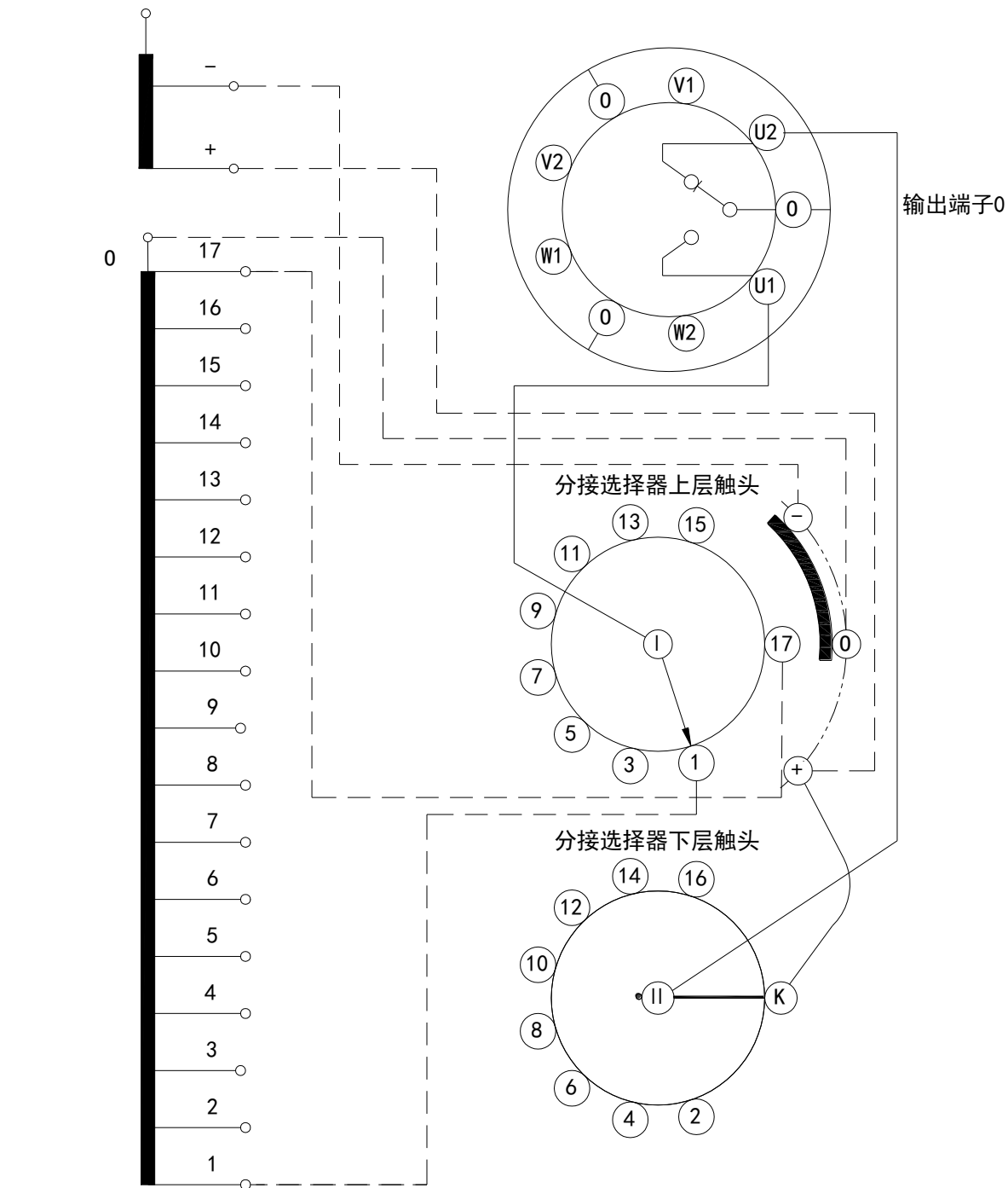
附图 63 VCM 型分接开关工作位置表和接线图 (18351G)
