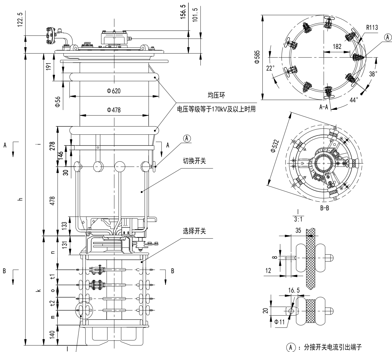
附图 10 VCM 型分接开关 I 800 不带极性选择器
