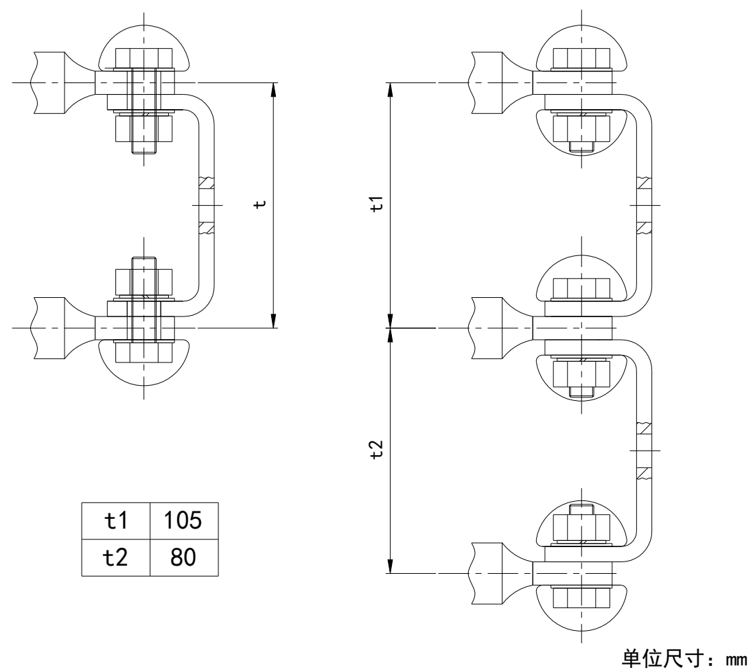
VCM型 I 800触头端子联接图
