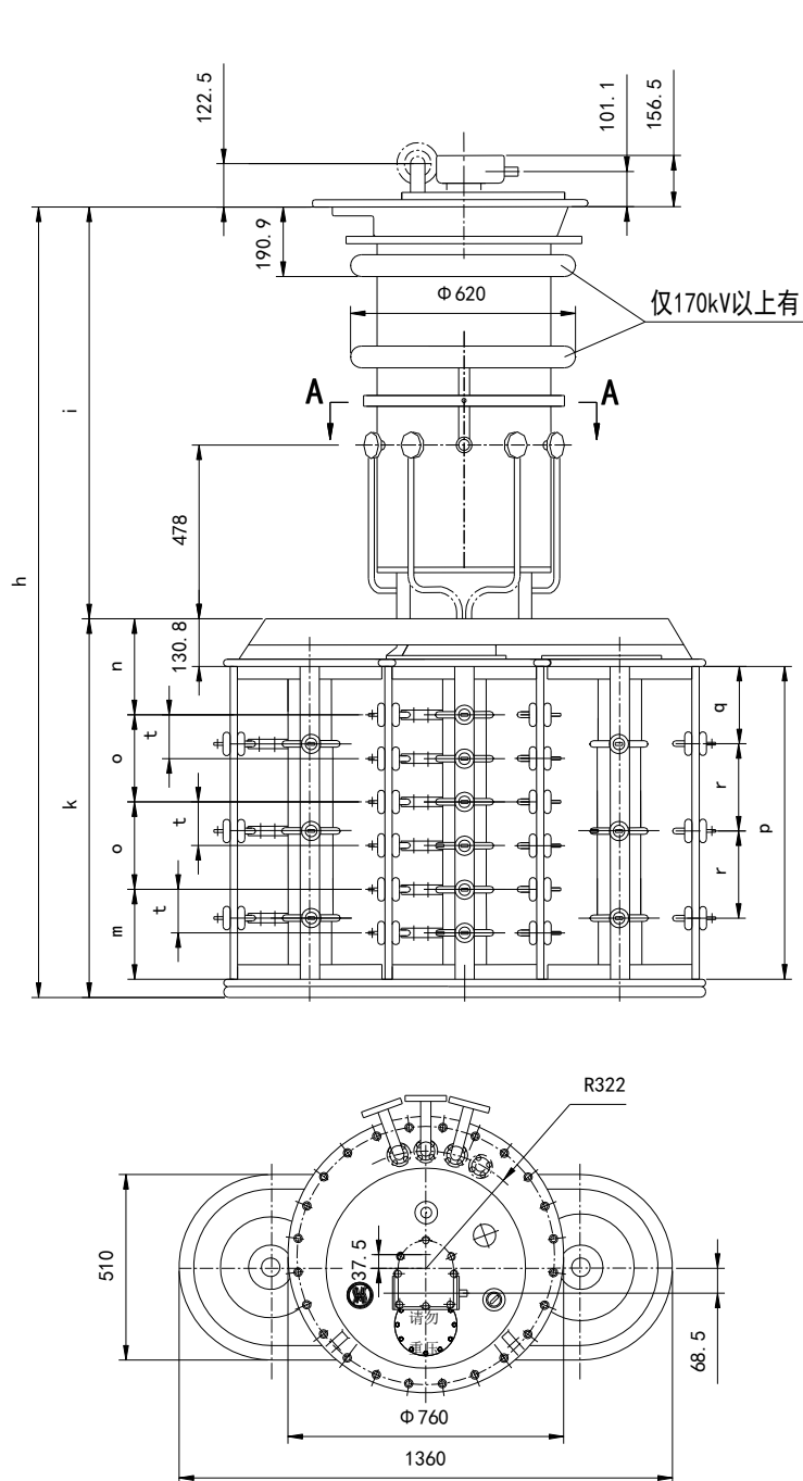
附图 31 VCM III 500Y/600Y 多级分接开关外形尺寸图
