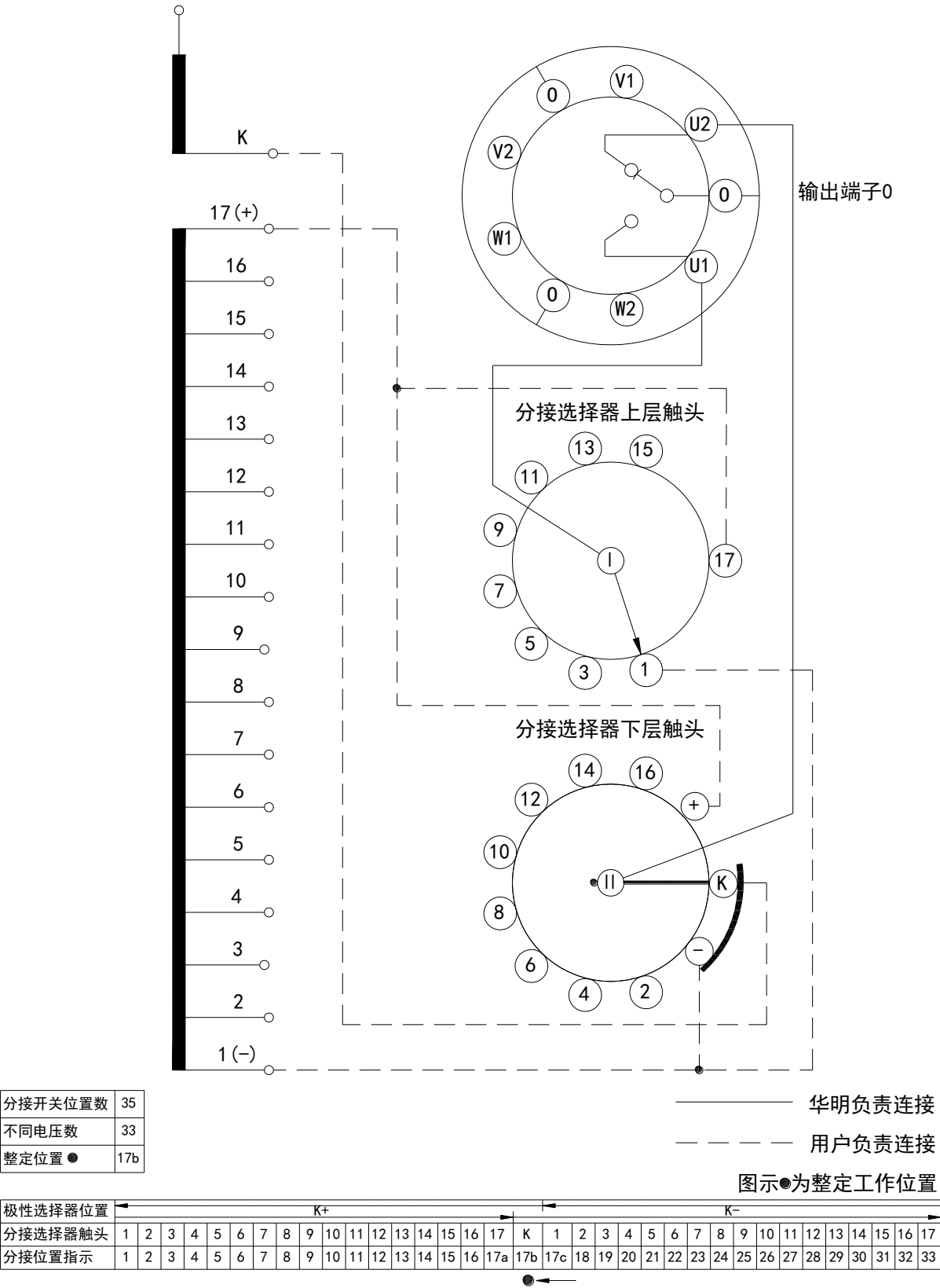
附图 66 VCM 型分接开关工作位置表和接线图 (18353W)
