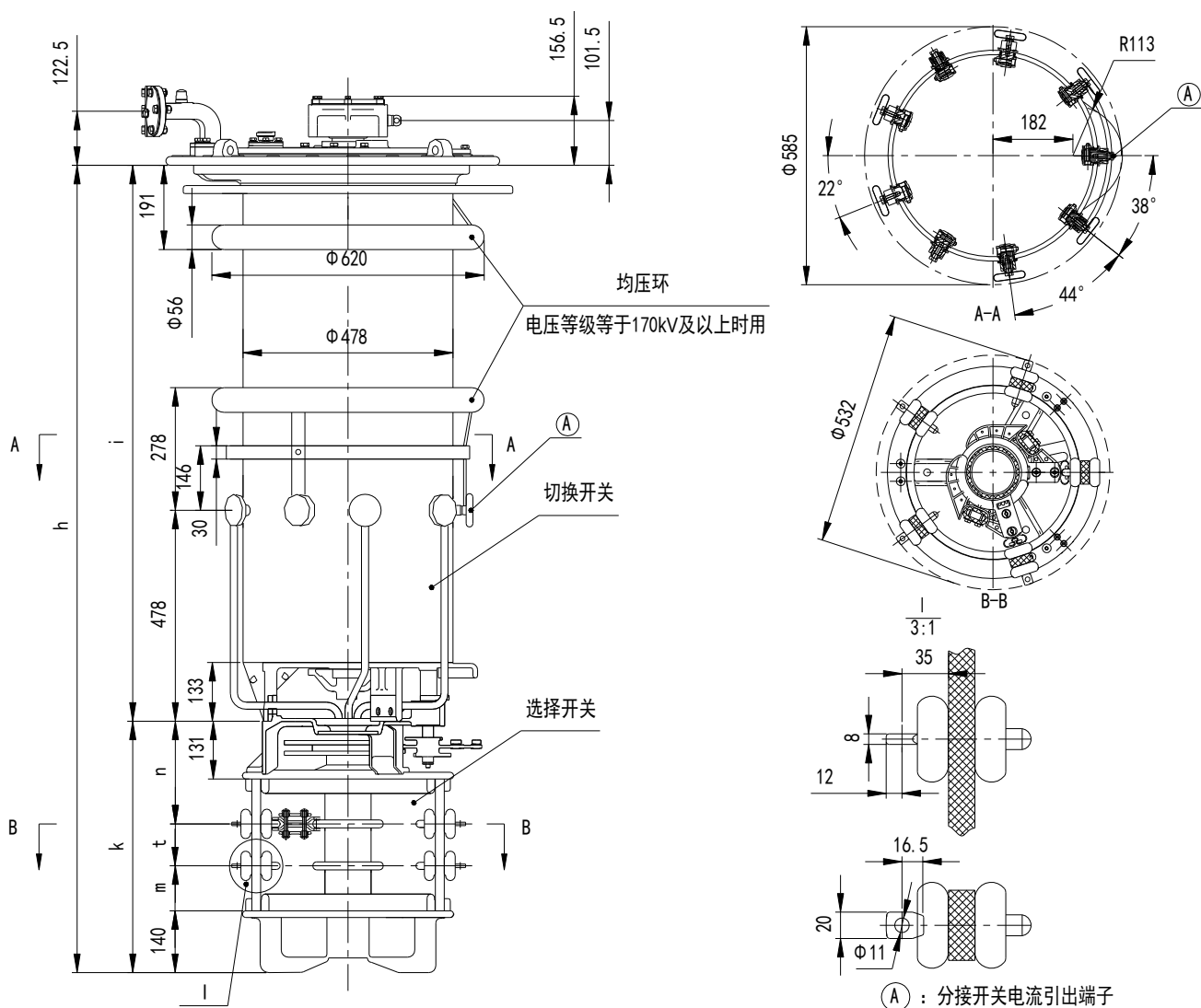
附图 7 VCM 型分接开关 I 500/600 不带极性选择器
