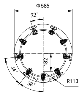
A-A剖视
