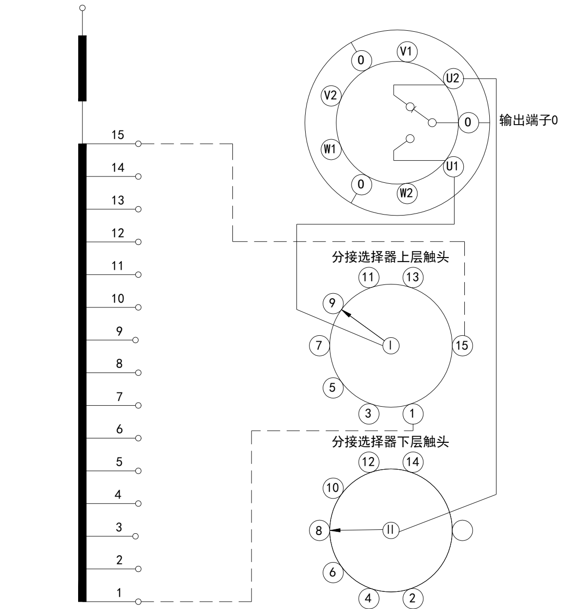
附图 55 VCM 型分接开关工作位置表和接线图 (16150)
