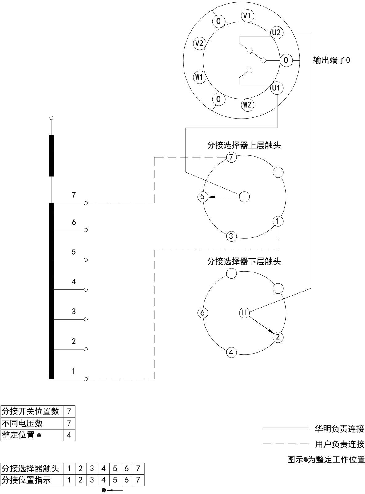
附图 35 VCM 型分接开关工作位置表和接线图 (10070)
