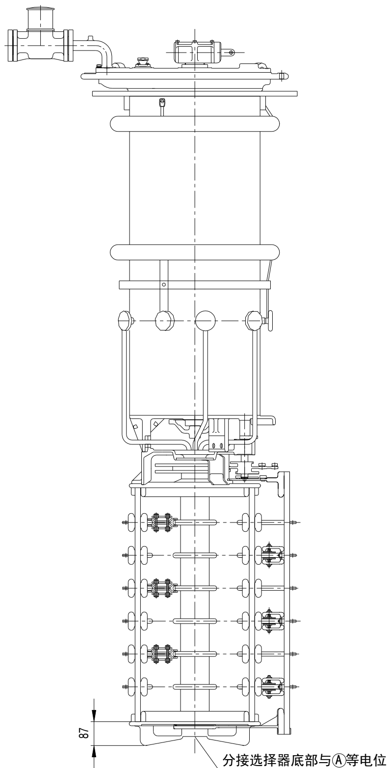
附图 17 VCM 型分接开关外形图 (配铝底座)
