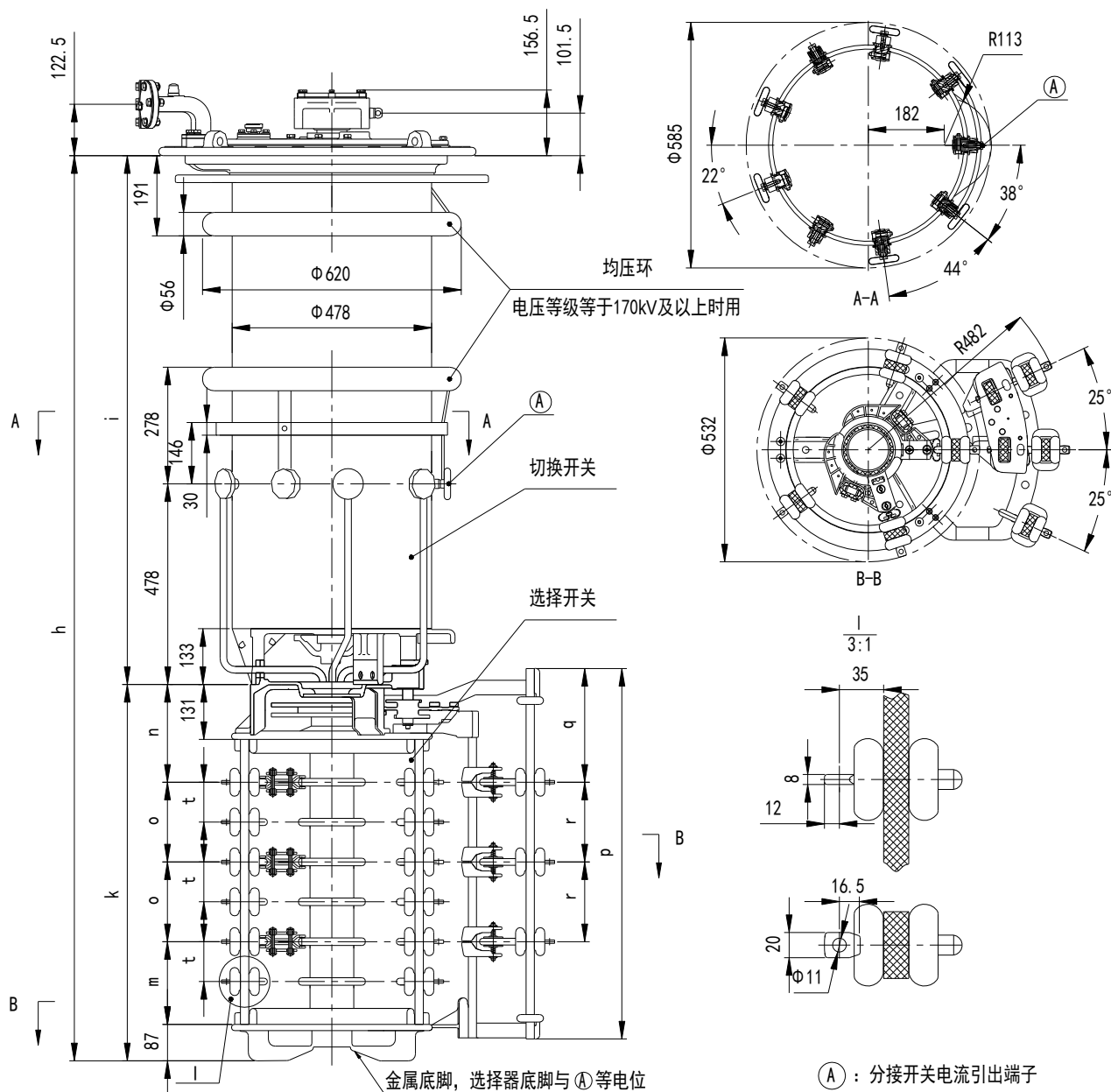
附图 3 VCM 型分接开关 III 500Y/600Y 带粗细调选择器
