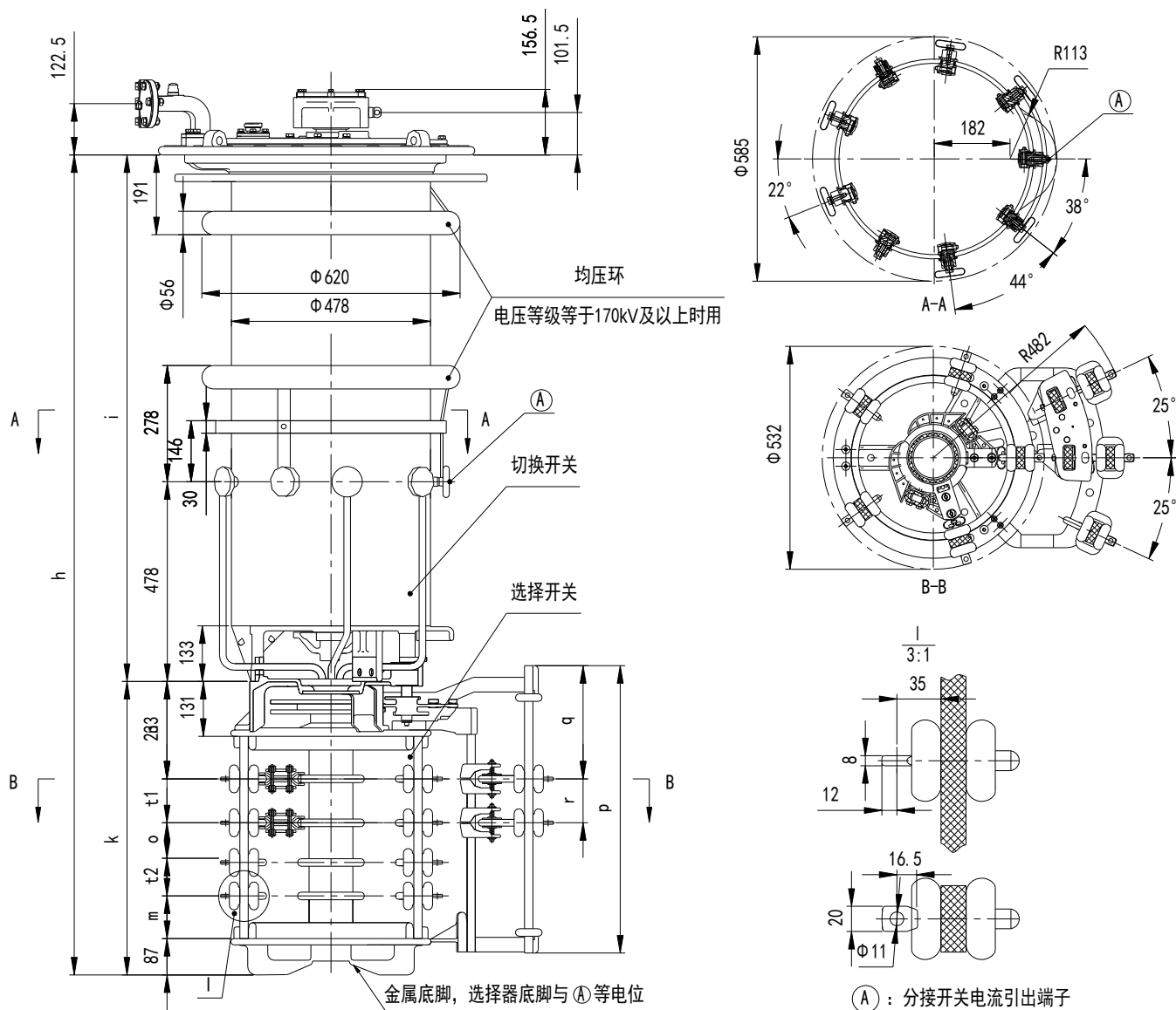
附图 12 VCM 型分接开关 I 800 带粗细调选择器
