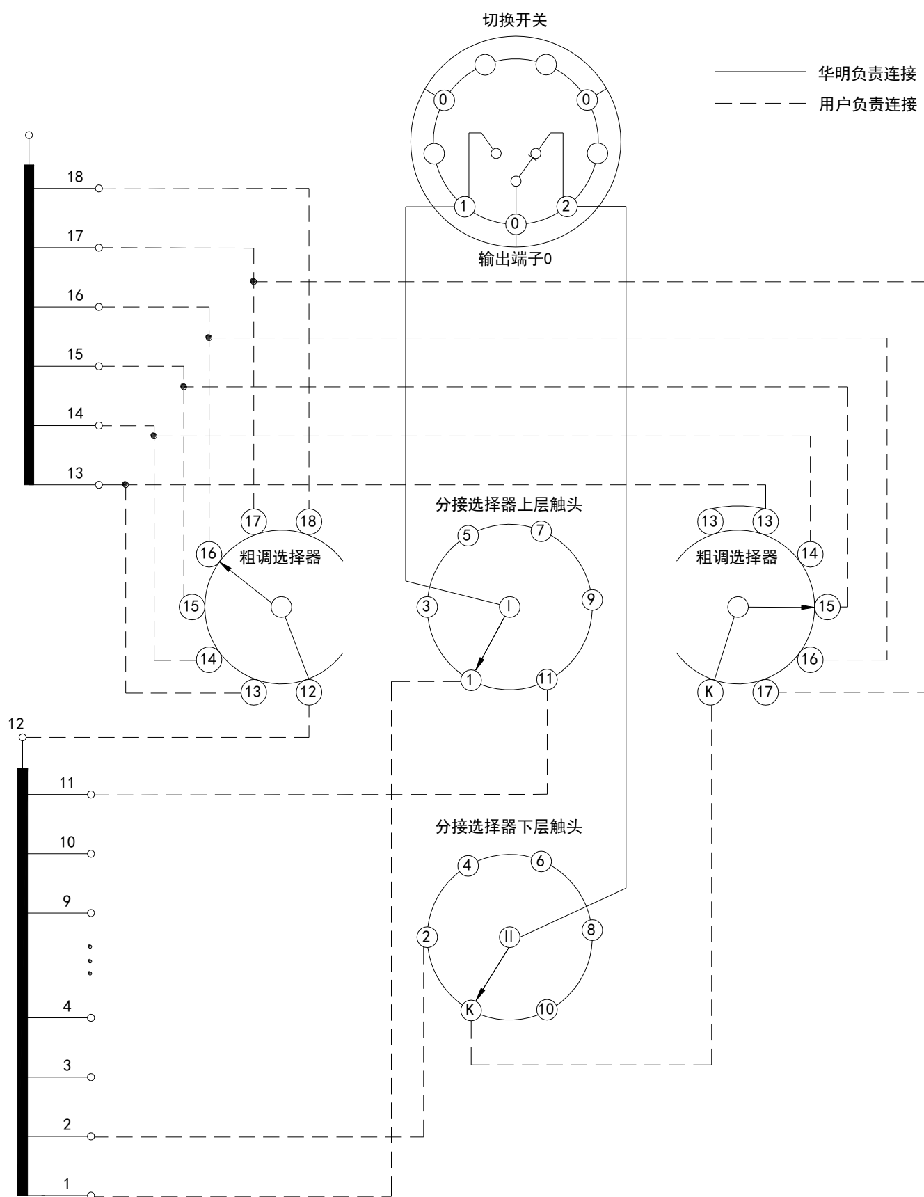
附图 69 12711G 档开关连接图
