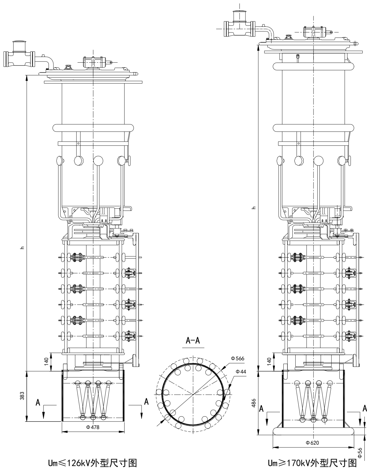
附图 16 VCM 型分接开关配电位电阻外形尺寸图
