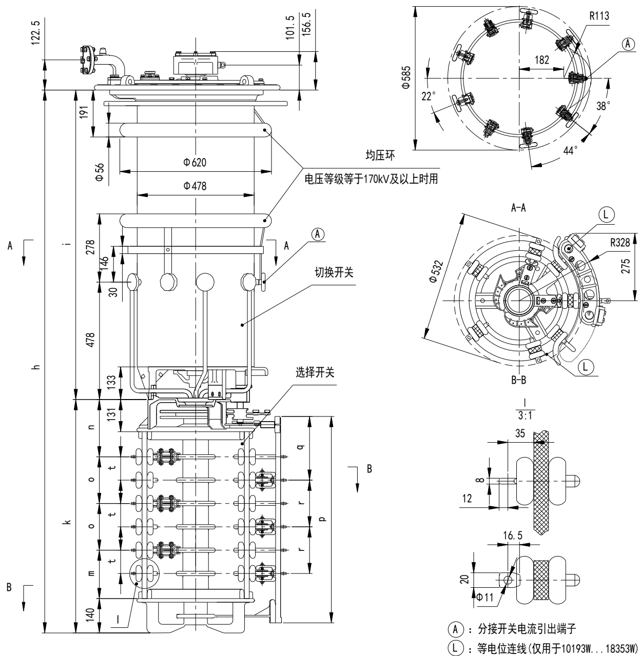
附图 2 VCM 型分接开关 III 500Y/600Y 带极性选择器
