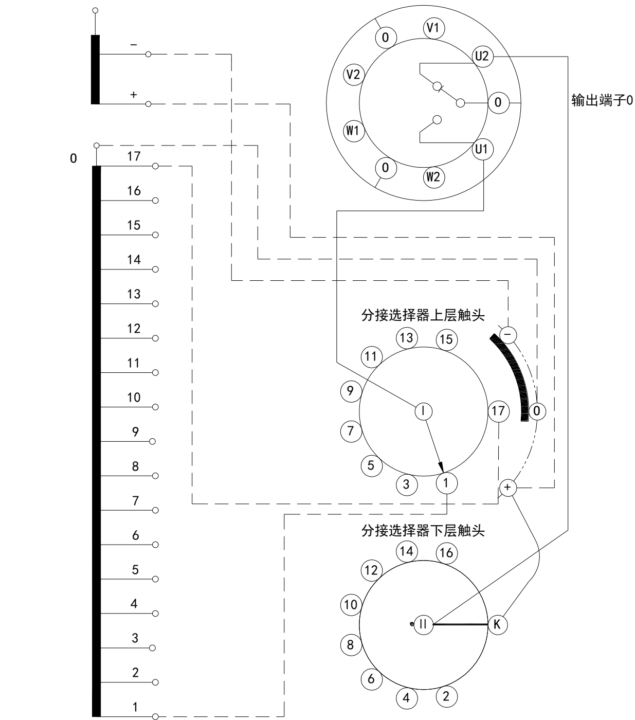
附图 65 VCM 型分接开关工作位置表和接线图 (18353G)
