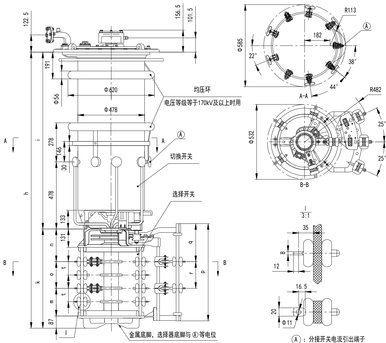
附图 6 VCM 型分接开关 II 500/600 带粗细调选择器
