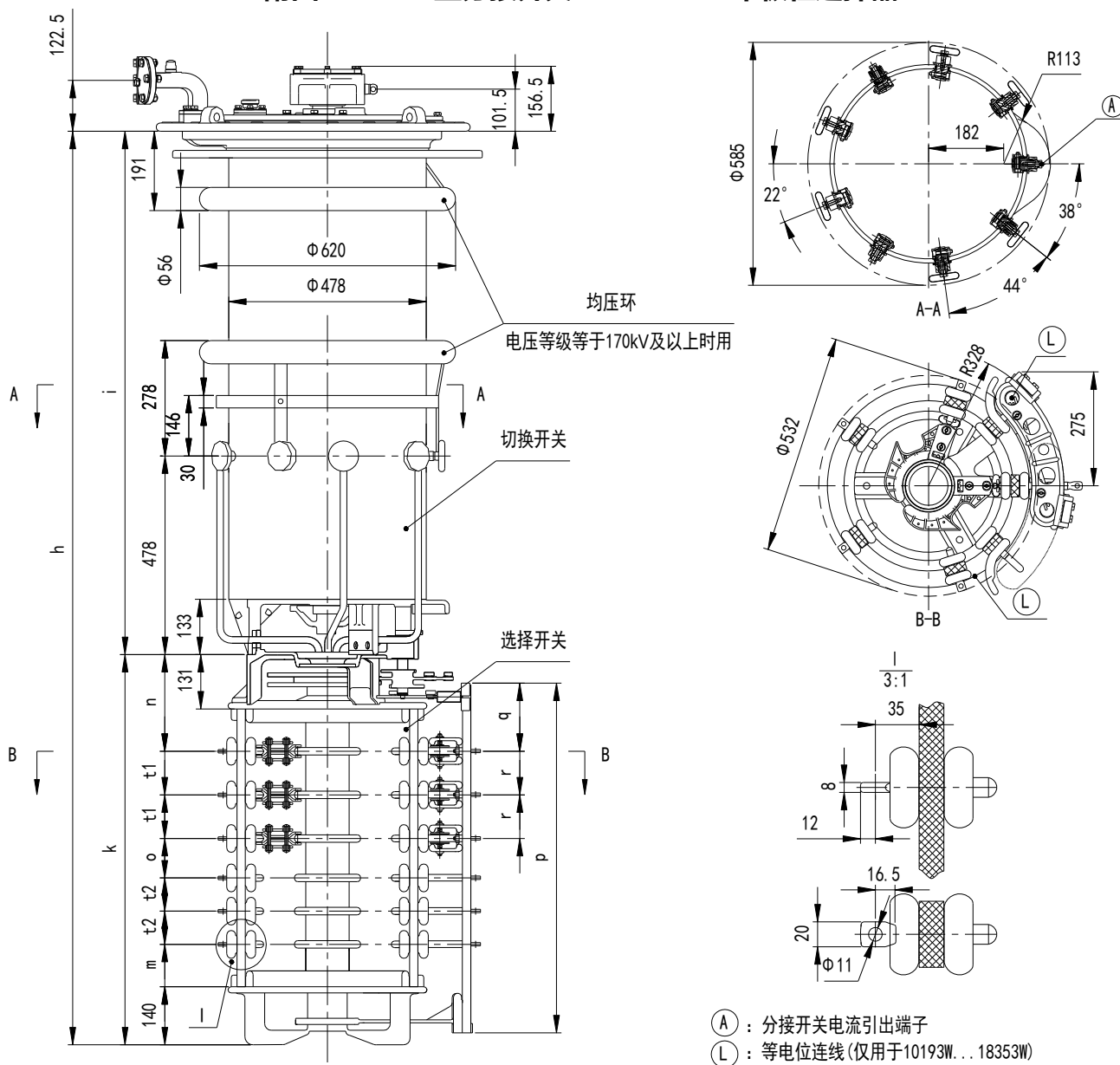
附图 14 VCM 型分接开关 I 1200/1500 带极性选择器
