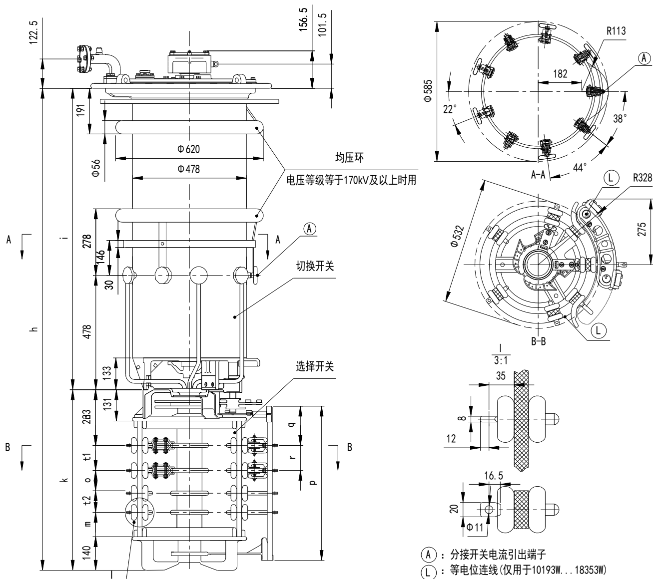
附图 11 VCM 型分接开关 1800 带极性选择器
