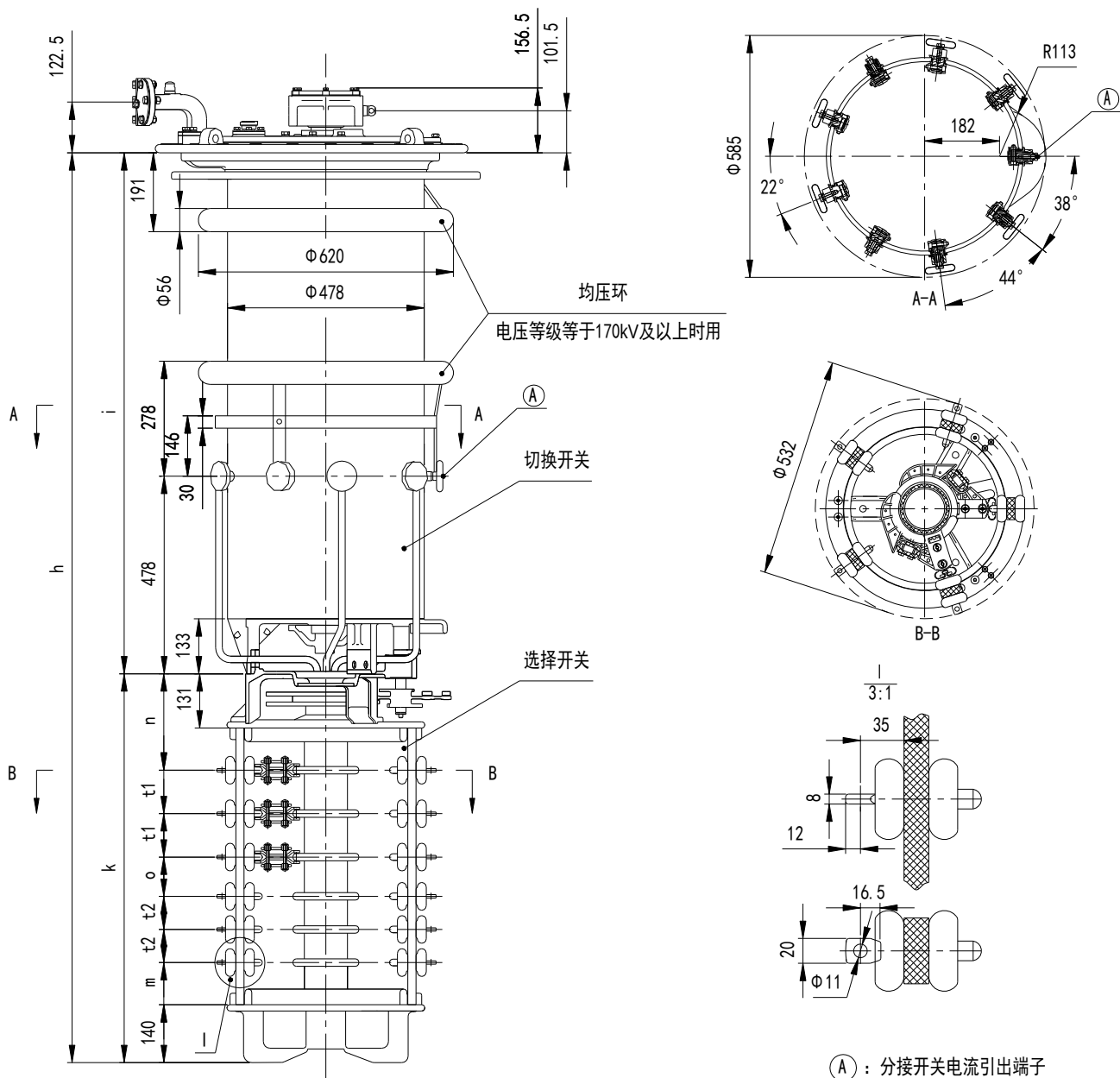
附图 13 VCM 型分接开关 I 1200/1500 不带极性选择器
