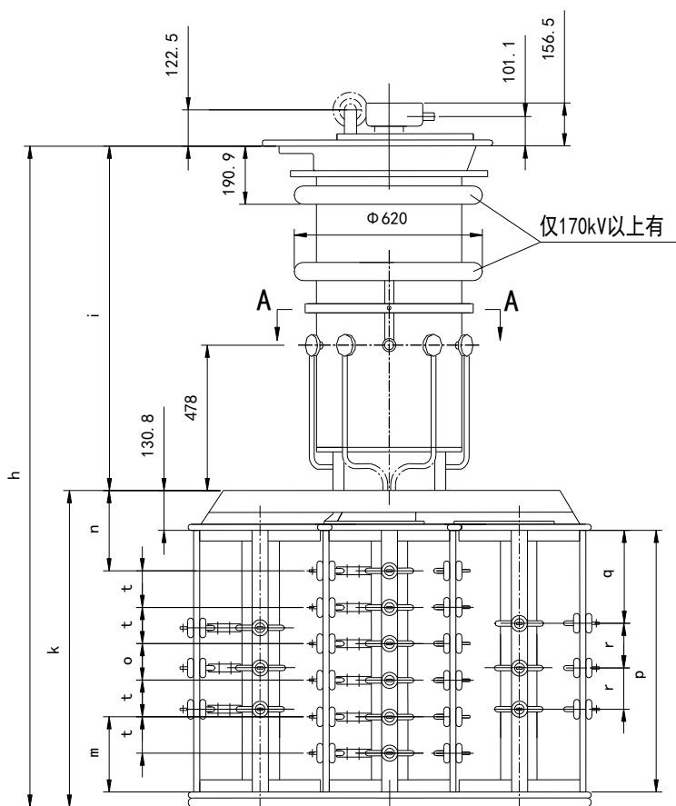
附图 34 VCM I 1200/1500 多级分接开关外形尺寸图
