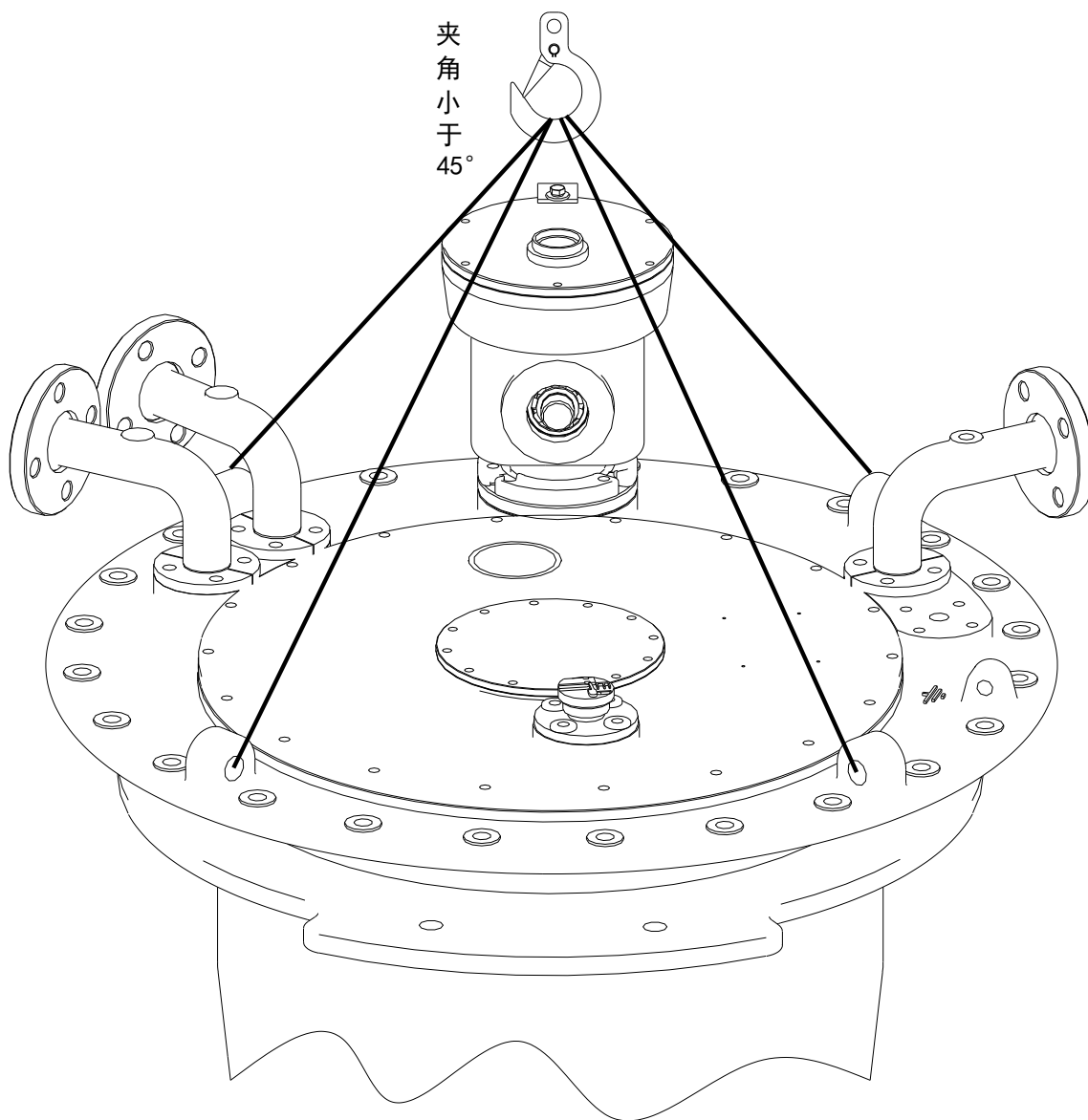
图 4-5 开关吊装图
