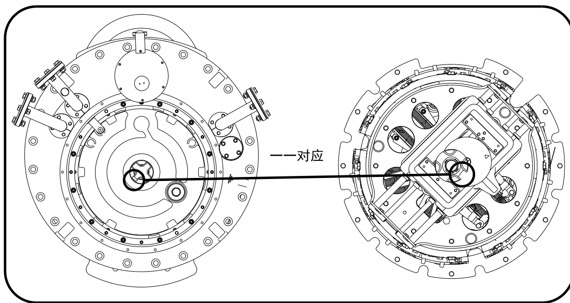
图 5-16 连接件的整定位置及法兰圈上的螺母固定
