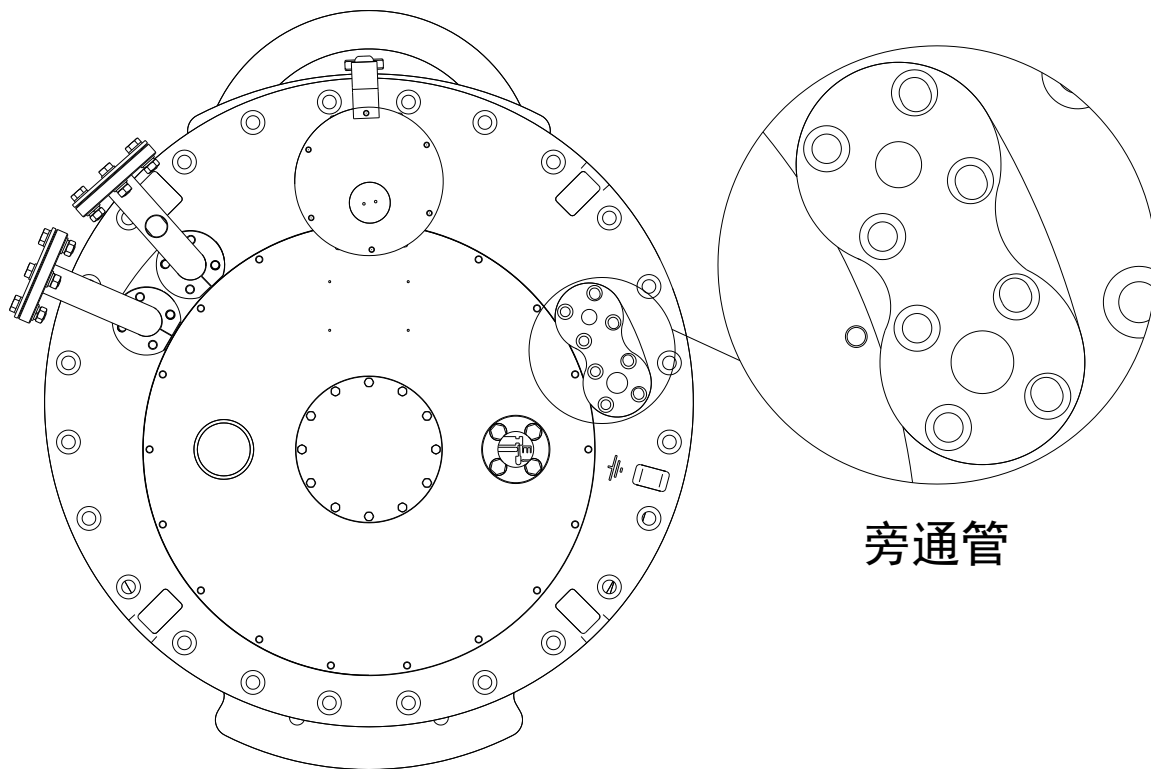
图 7-2 管接头在开关头上的位置
